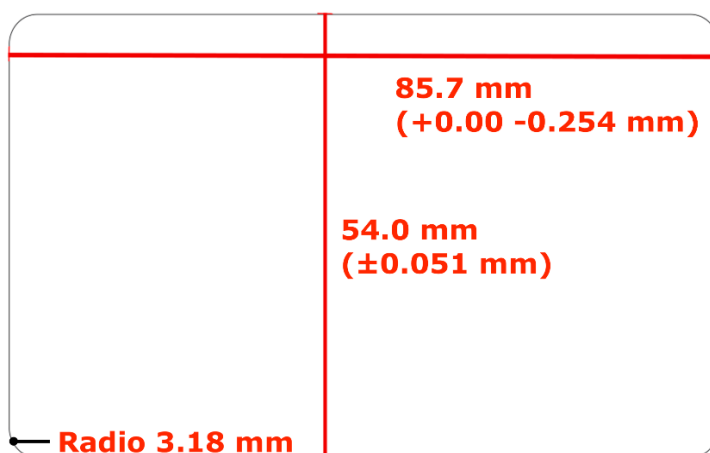
Figura 1. Dimensiones de Monedero SINPE-TP
