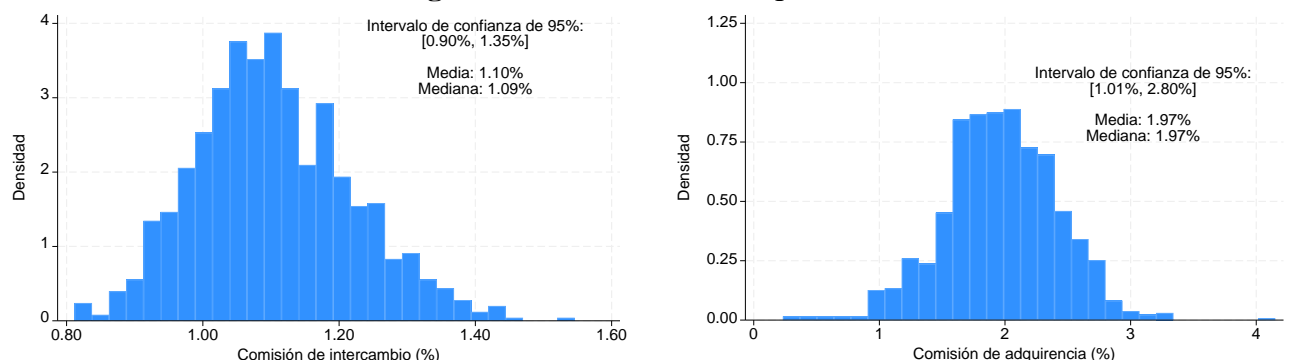
Figura 5. Distribución de las comisiones de adquirencia e intercambio según el método de Bootstrap
