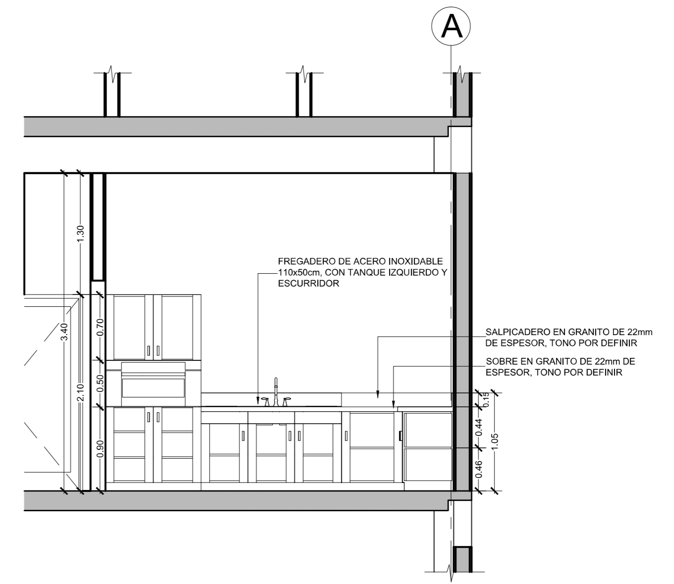
DETALLE COCINA TERCER NIVEL (M-01)
