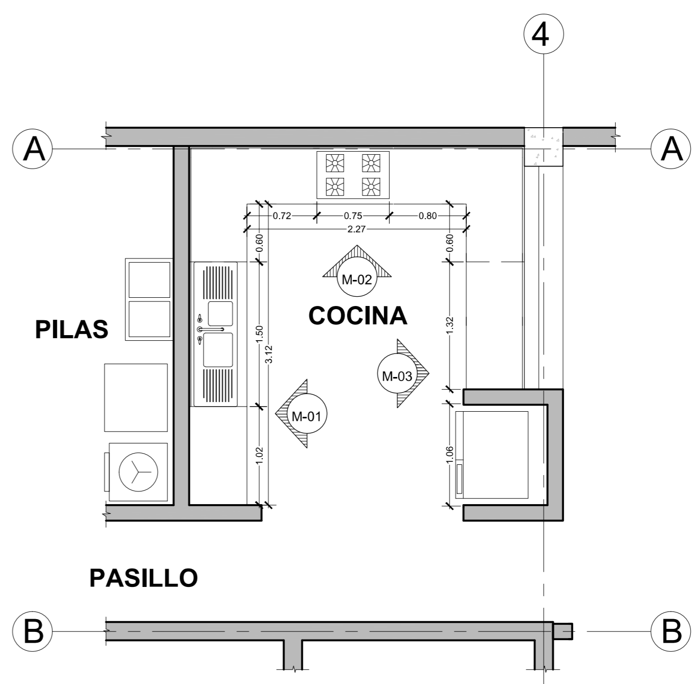
DETALLE COCINA TERCER NIVEL (PLANTA)
