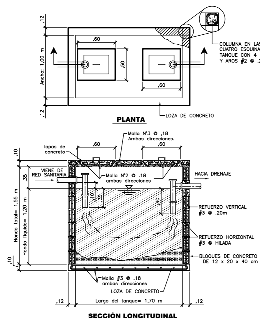
DETALLE DEL TANQUE SEPTICO SIN ESCALA
