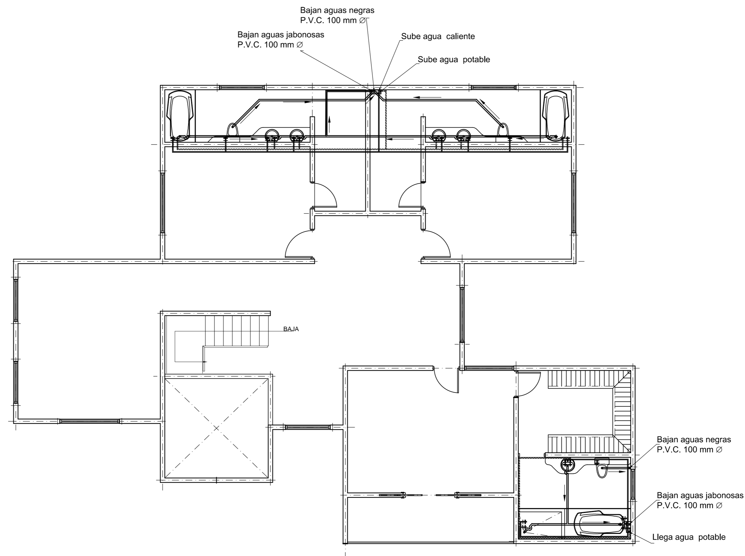
PLANTA DE OBRA MECANICA. AGUAS NEGRAS, AGUAS JABONOSAS Y AGUA POTABLE SEGUNDO NIVEL
