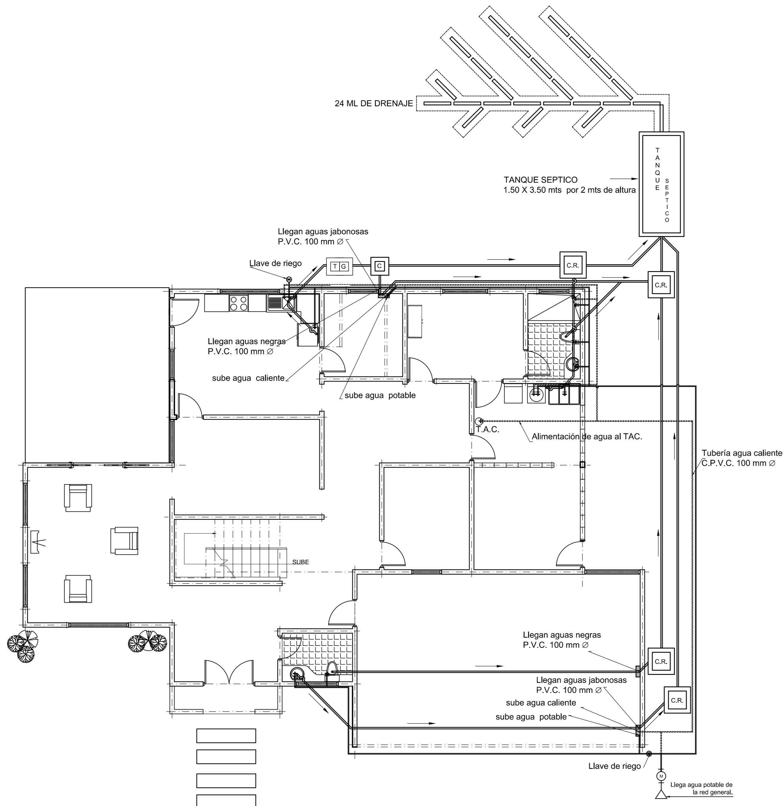
PLANTA DE OBRA MECANICA. AGUAS NEGRAS, AGUAS JABONOSAS Y AGUA POTABLE PRIMER NIVEL
