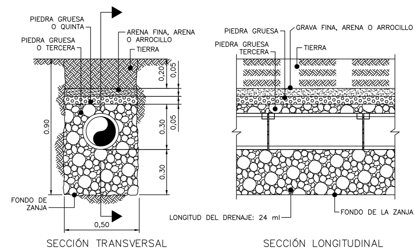
DETALLE DE DRENAJE SIN ESCALA
