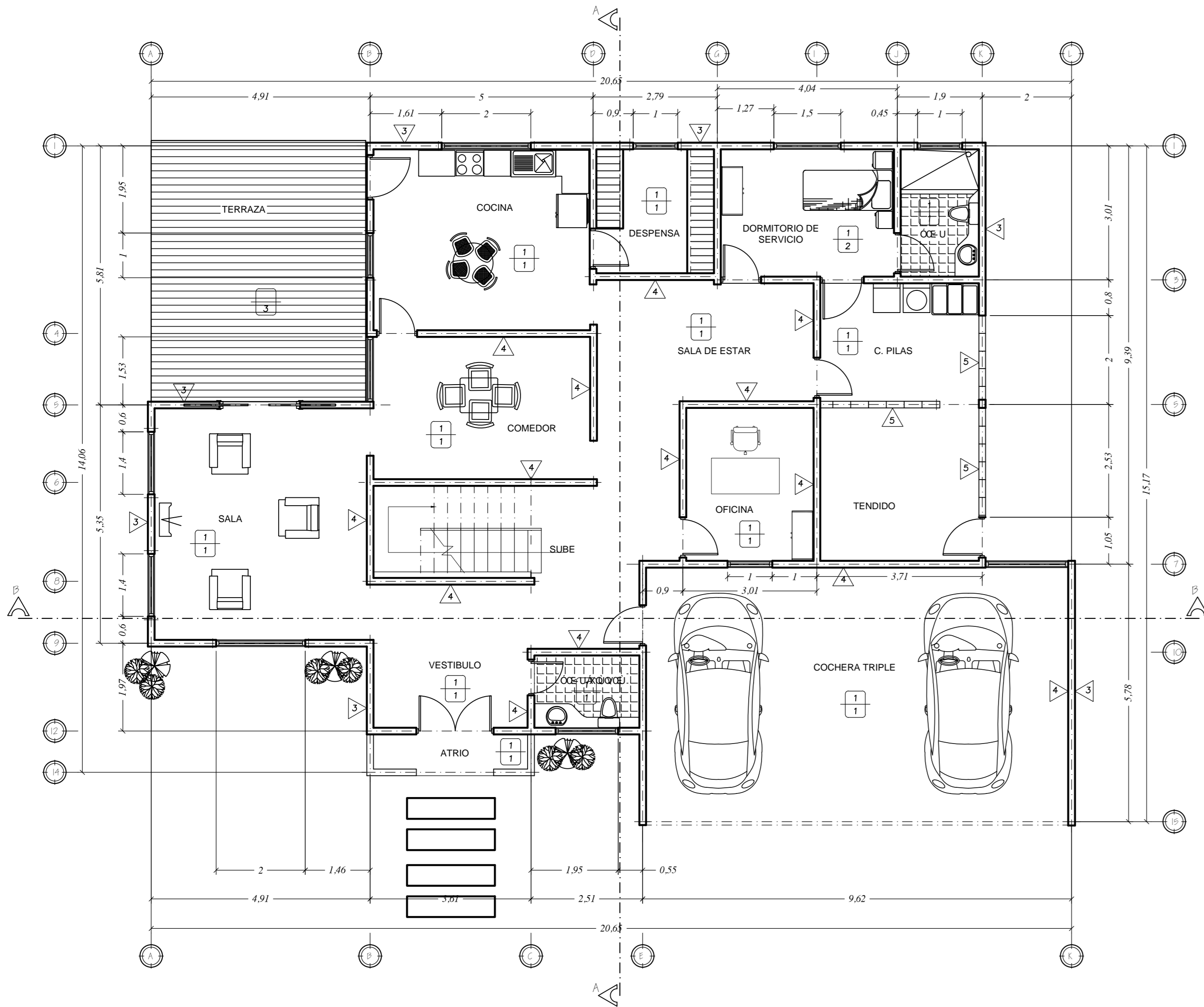
PLANTA DE DISTRIBUCION ARQUITECTONICA PRIMER NIVEL
