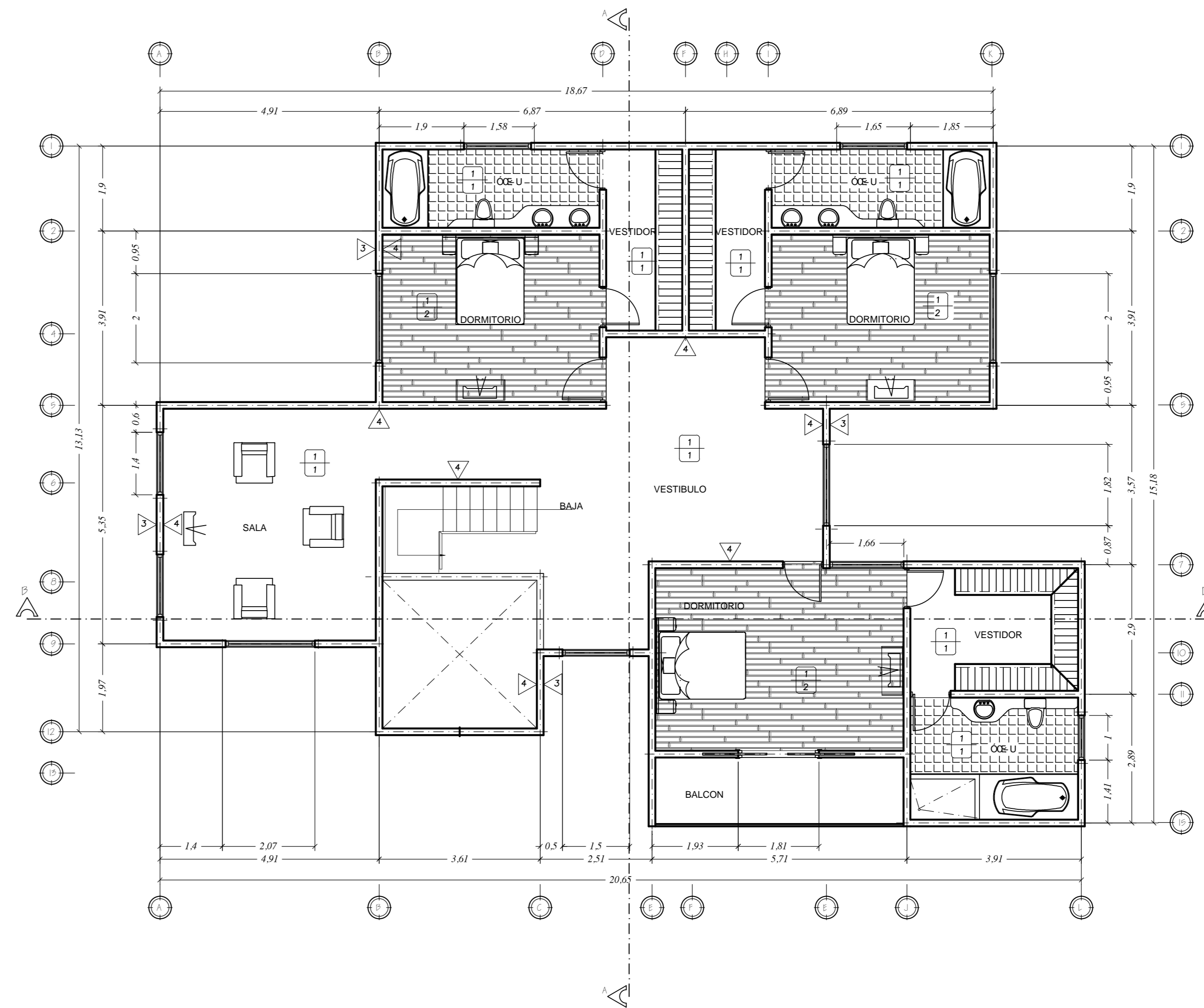
PLANTA DE DISTRIBUCION ARQUITECTONICA SEGUNDO NIVEL
